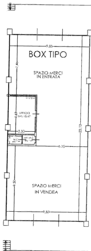
BOX TIPO
