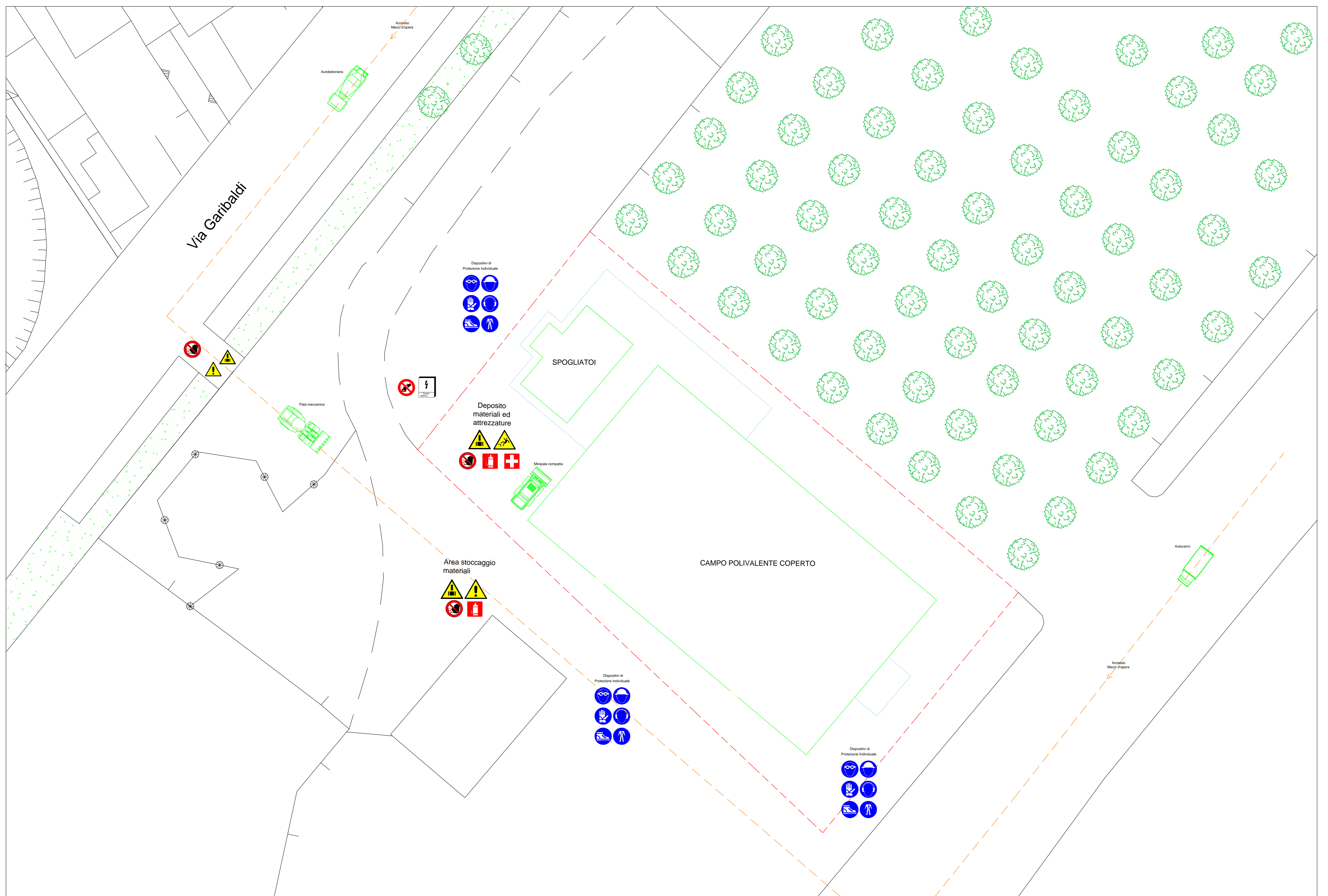
PLANIMETRIA DI CANTIERE
